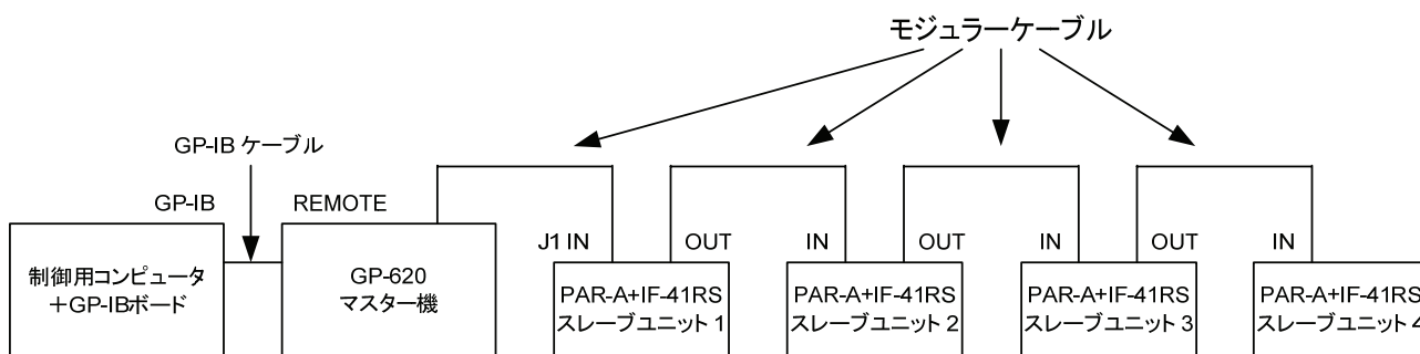
Fig.15 GP-620 を使用したりモートコントロール
