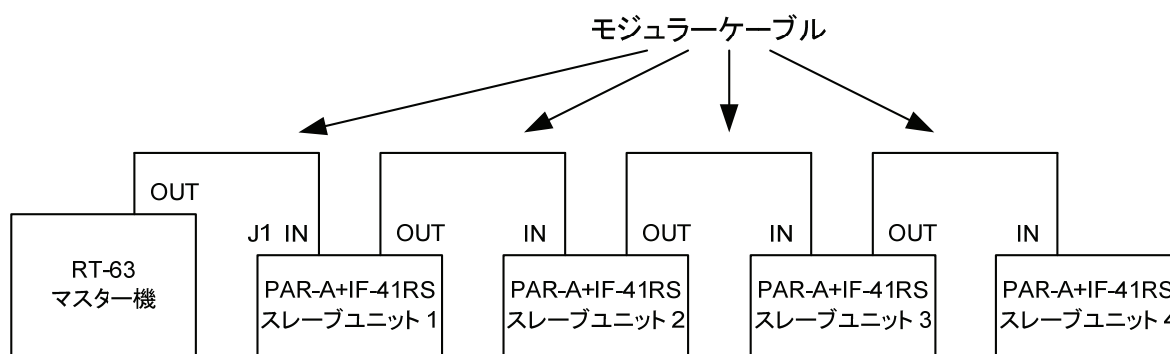
Fig.14 RT-63 を使用したりモートコントロール
